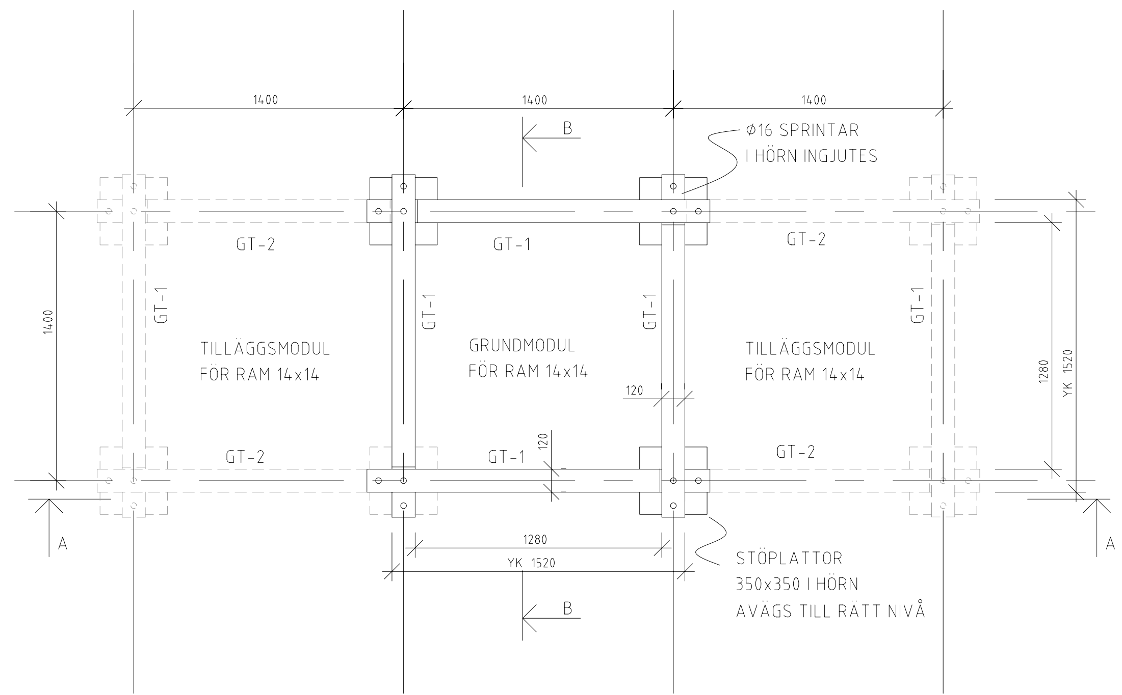
PLAN 1:20 TRÄDGRÖP MODUL 14x14 I PREFAB-BETONG
