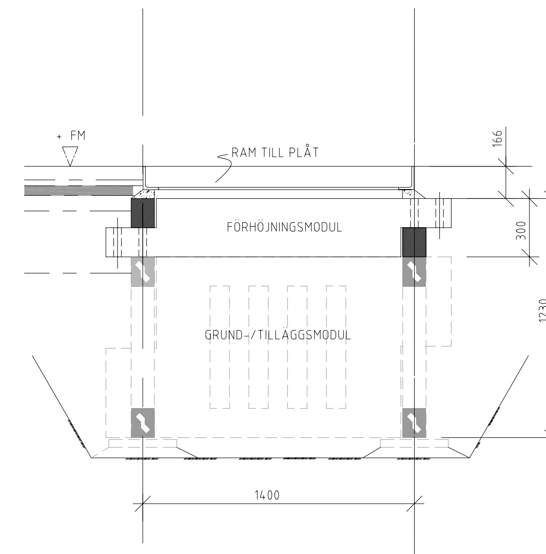
B 1:20 PRINCIP MED FÖRHÖJNINGSMODUL
