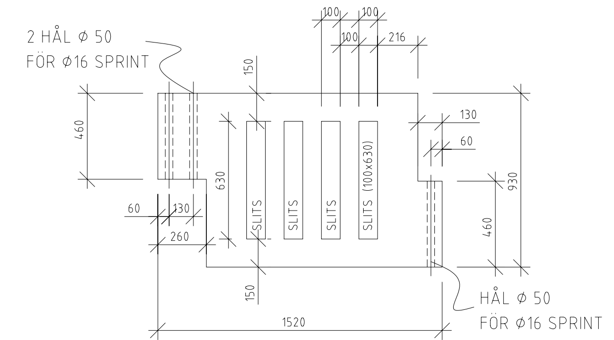
GT-2 TILLÄGGSMODUL FÖR RAM 14x14 fj=120 MÄTTSÄTTNING
