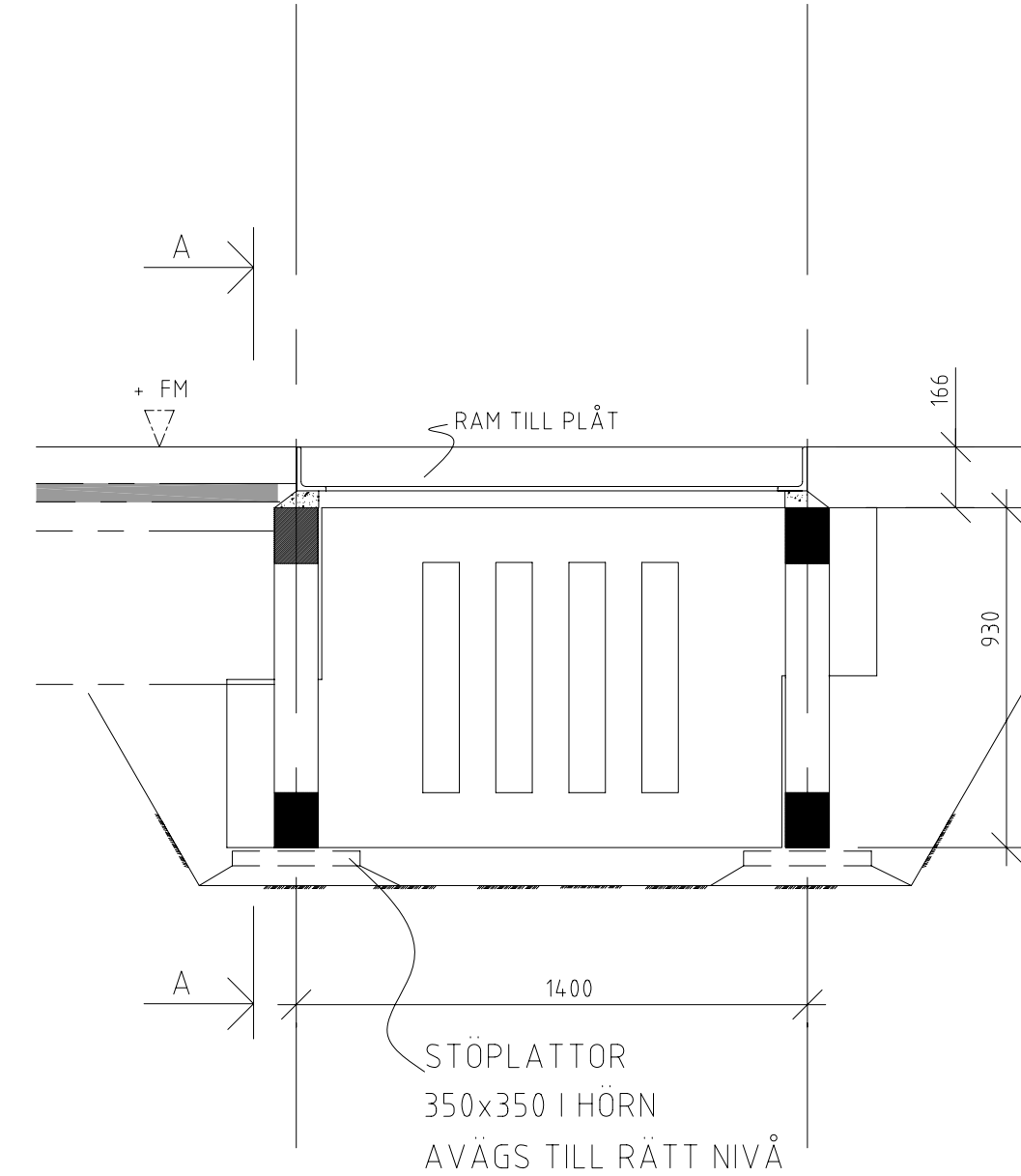
B 1:20 GRUNDMODUL
