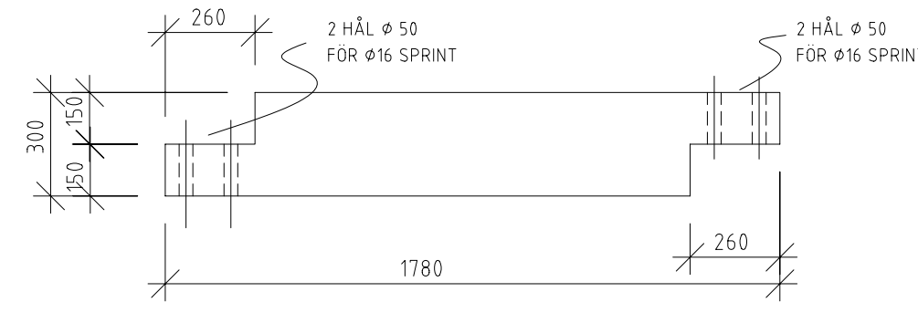
GT-1FH 1:20
