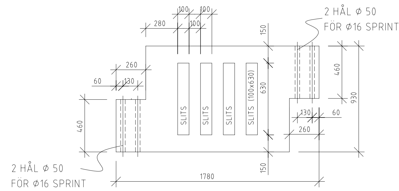
GT-1 GRUNDMODUL FÖR RAM 14x14 fj=120 MÄTTSÄTTNING
